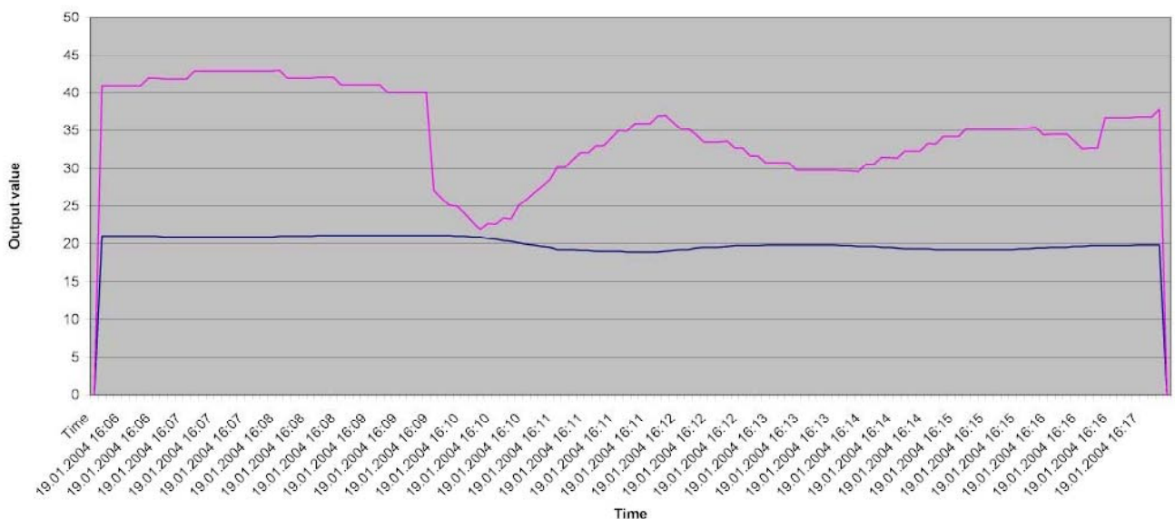
Relevé de la température de soufflage sur l'ACS700
