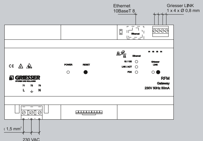
Schéma de raccordement RFM
